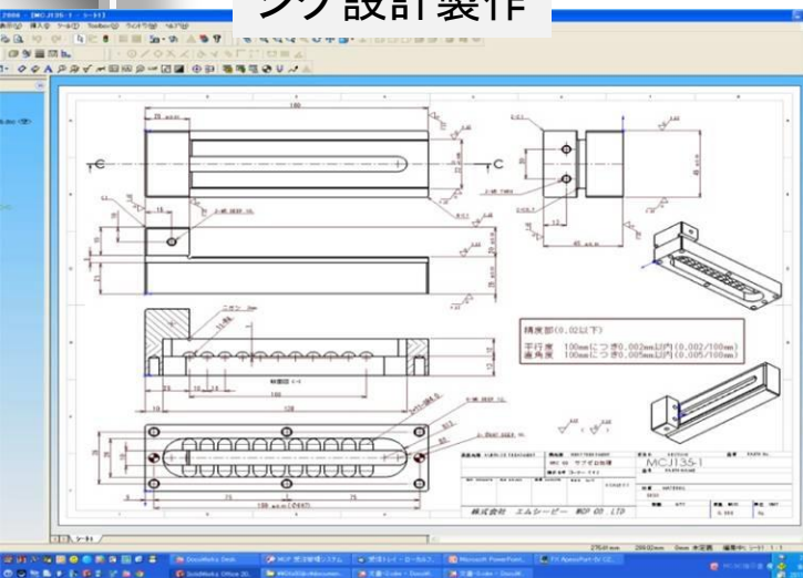
ジグ設計製作
